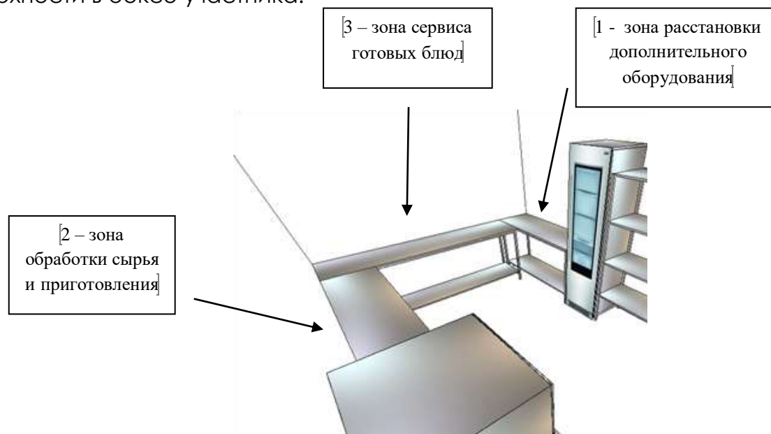
Рисунок 2 – Примерная схема организации рабочей поверхности участника в боксе
